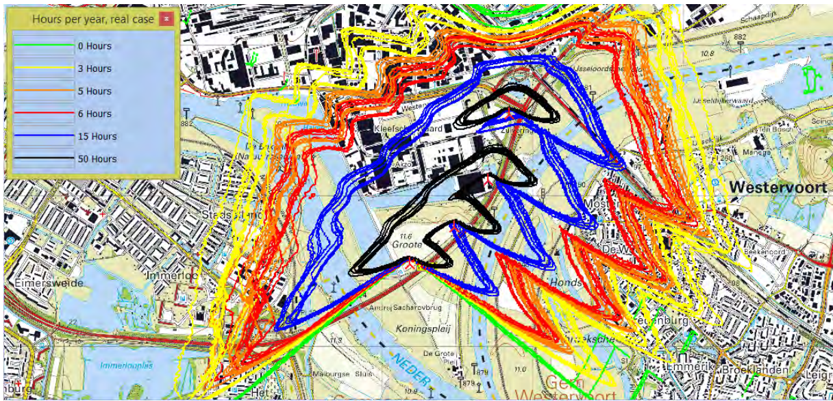
Figuur 4a: Vergelijking slagschaduwcontouren voor alle turbinetypen (uren per jaar)
